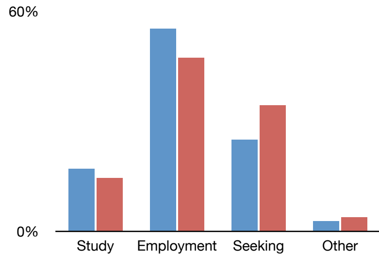
Comp sci
