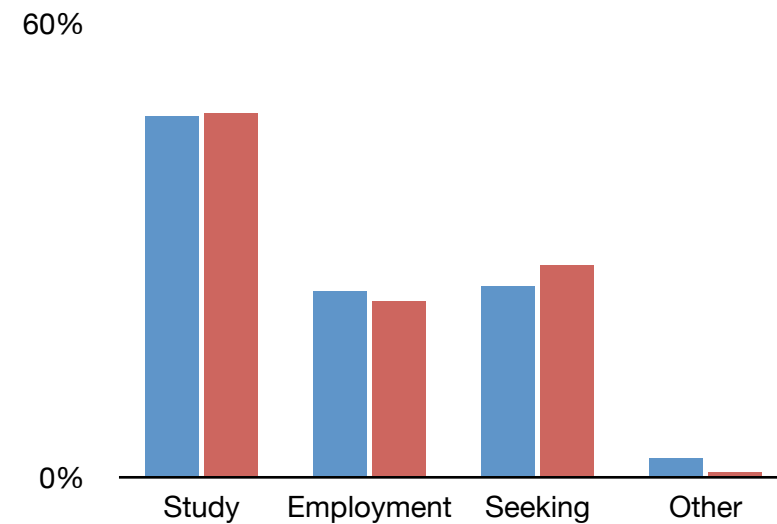
Geosci
